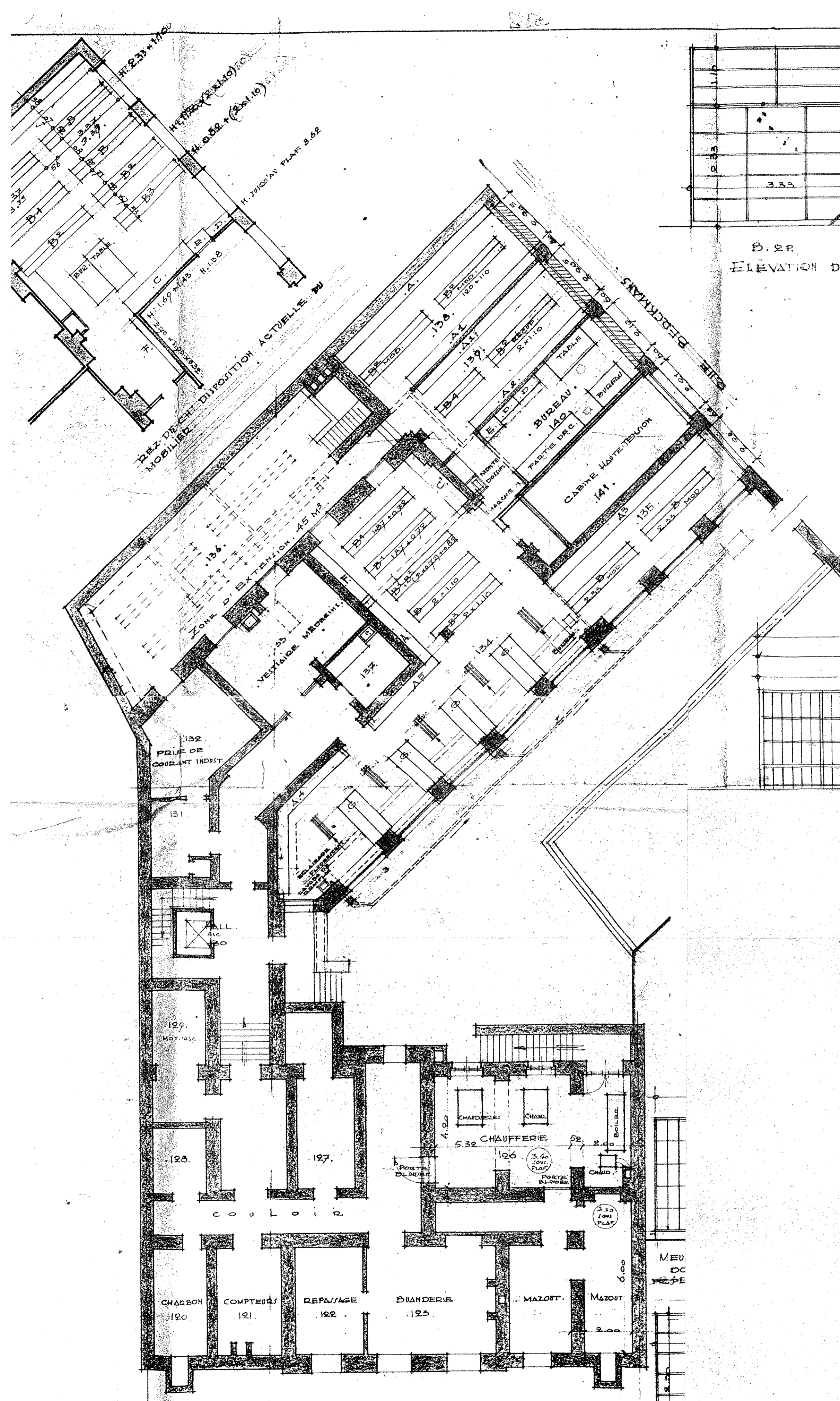
PLAN DU SOUS-SOL.
