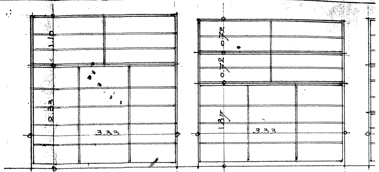
B. 2 P. ELEVATION DU MOBILIER ACTUEL, AVEC SES COMPC
